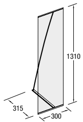
VA 8313 300 x 1310 mm
